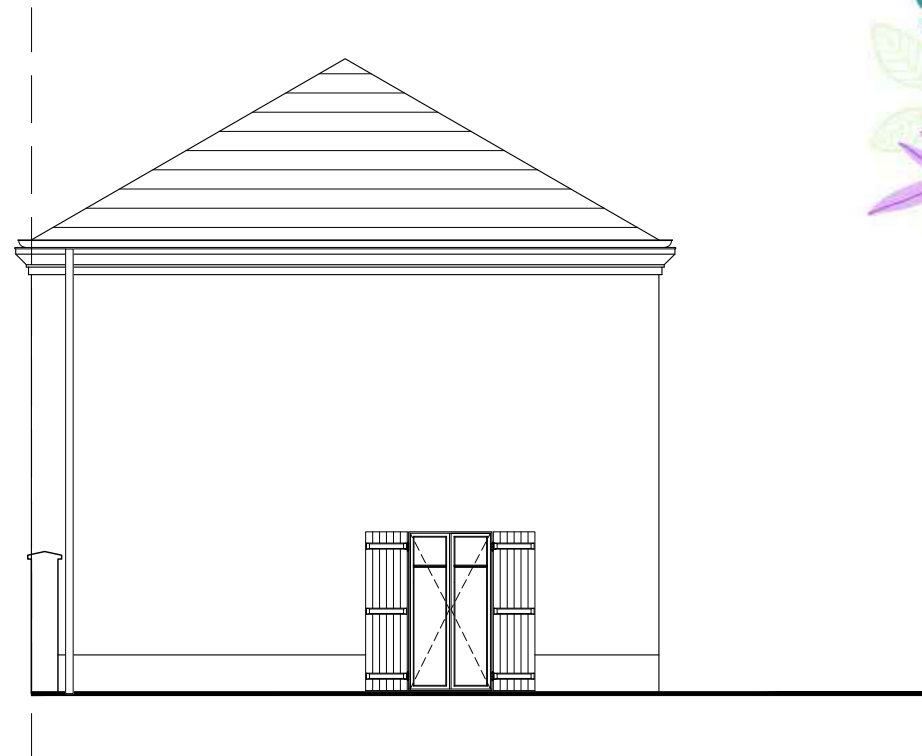
FACADE LATERALE NORD
