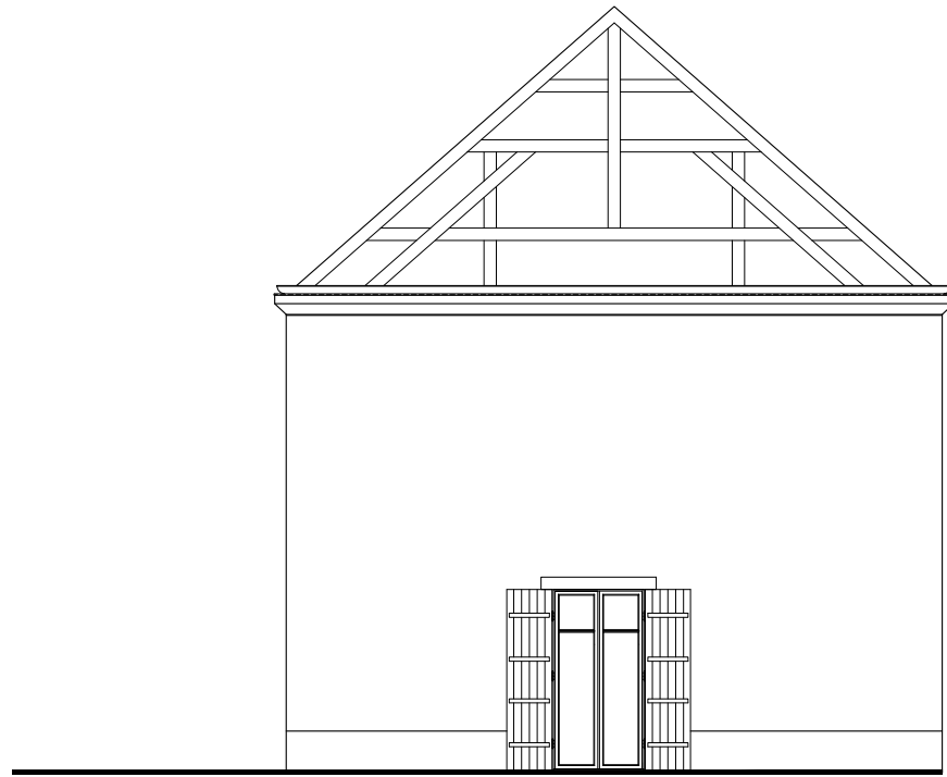
FACADE LATÉRALE SUD
