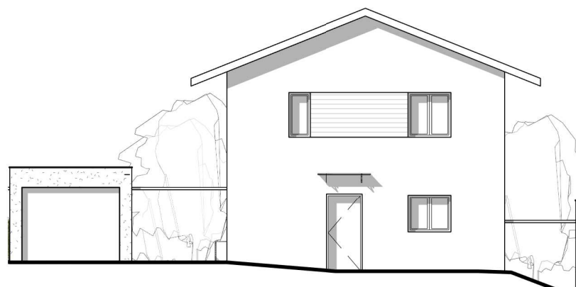
FACADE NORD
